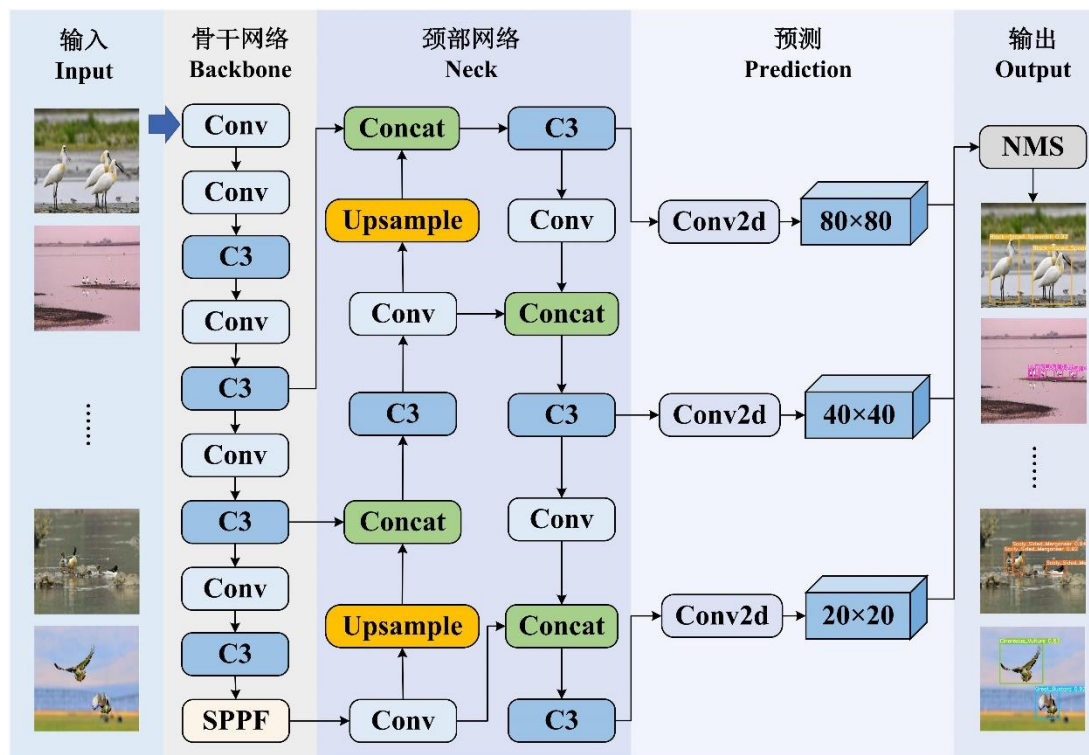
附录 1 YOLOv5s 模型结构。Upsample: 最近邻插值上采样。
