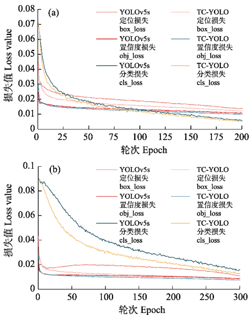
附录 2 数据集 Beijing-28 (a)与 CUB200-2011 (b)损失函数对比图
