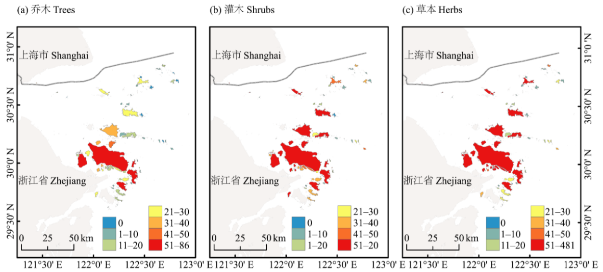
附录 4 舟山群岛 92 个岛屿不同生长型植物丰富度的空间分布。(a)乔木; (b)灌木; (c)草本。
