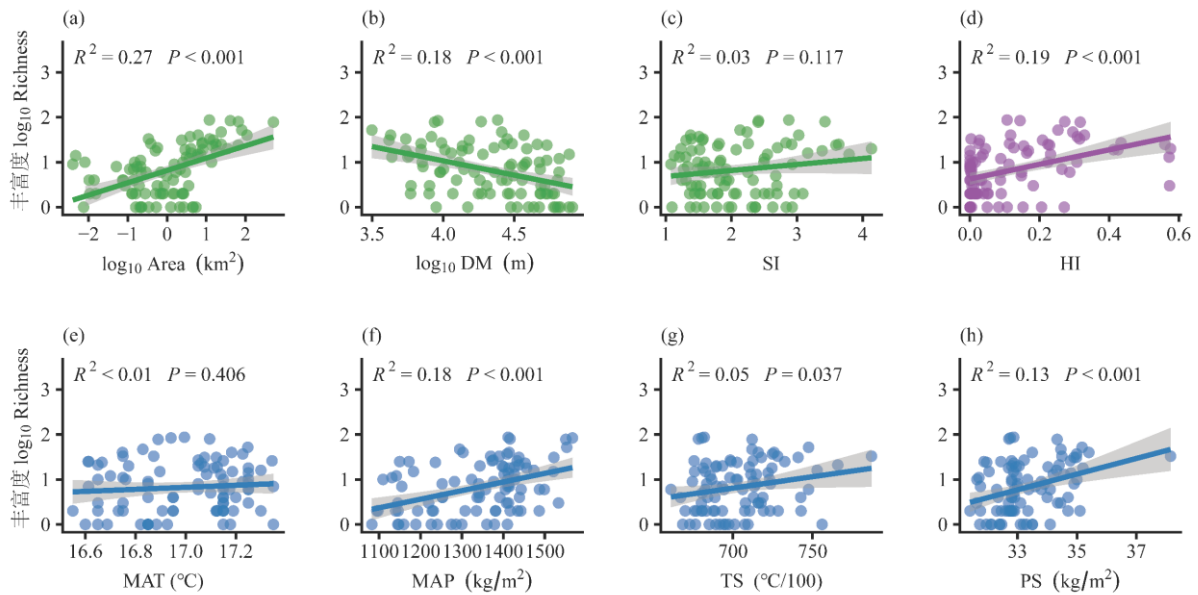
附录 5 乔木丰富度与环境因子的相关性。(a)面积(Area);(b)距大陆距离(DM);(c)岛屿形状指数(SI);(d)人类影响指数(HI);(e)年均温(MAT);(f)年降水量(MAP);(g)温度季节性(TS);(h)降水季节性(PS)。
