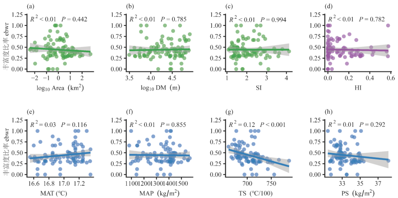
附录 10 常绿阔叶木本植物比率与环境因子的相关性。(a)面积(Area);(b)距大陆距离(DM);(c)岛屿形状指数(SI);(d)人类影响指数(HI);(e)年均温(MAT);(f)年降水量(MAP);(g)温度季节性(TS);(h)降水季节性(PS)。
