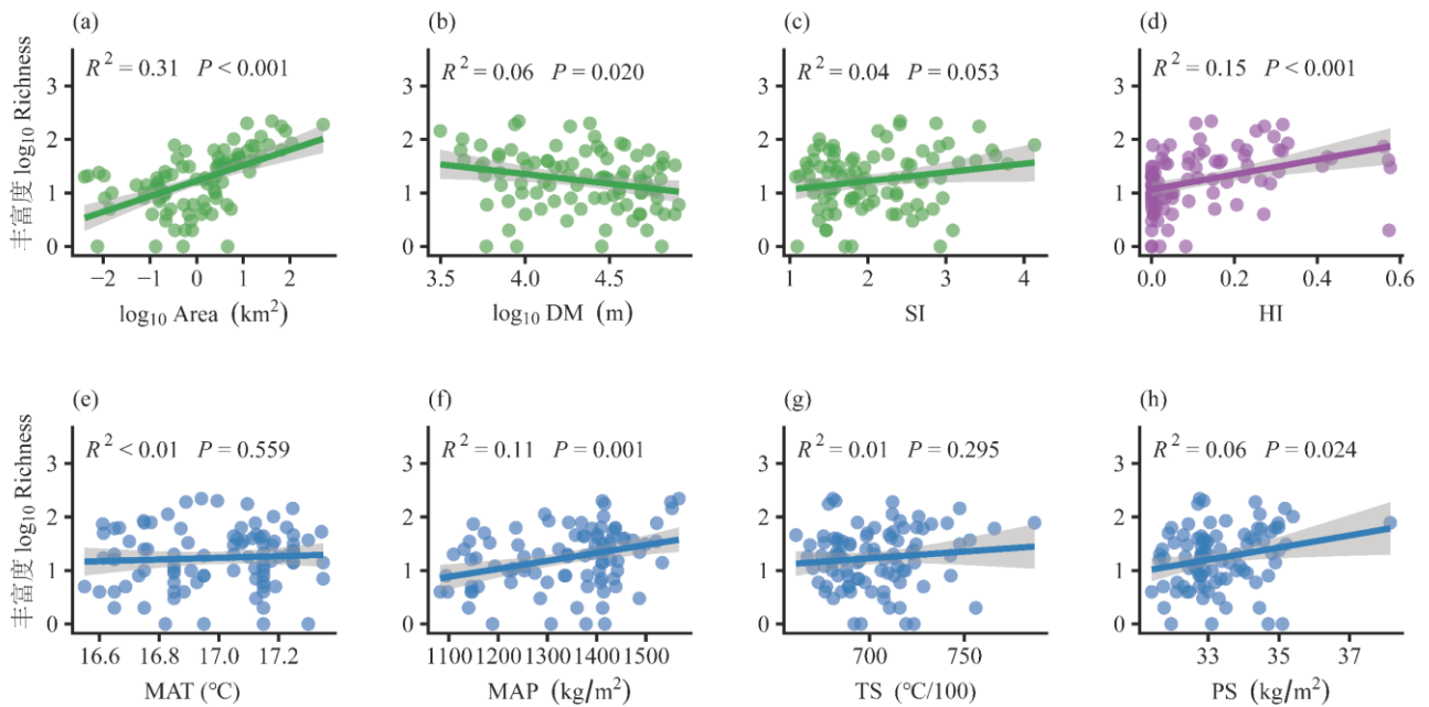
附录 6 灌木丰富度与环境因子的相关性。(a)面积(Area);(b)距大陆距离(DM);(c)岛屿形状指数(SI);(d)人类影响指数(HI);(e)年均温(MAT);(f)年降水量(MAP);(g)温度季节性(TS);(h)降水季节性(PS)。
