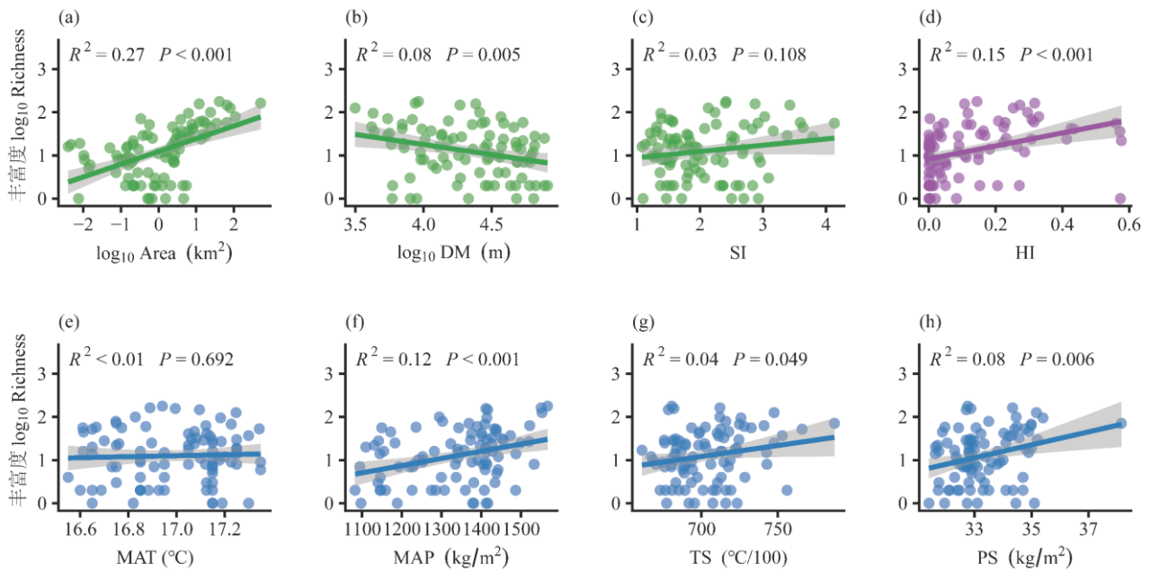
附录 9 落叶阔叶木本植物丰富度与环境因子的相关性。(a)面积(Area); (b)距大陆距离(DM); (c)岛屿形状指数(SI); (d)人类影响指数(HI); (e)年均温(MAT); (f)年降水量(MAP); (g)温度季节性(TS); (h)降水季节性(PS)。
