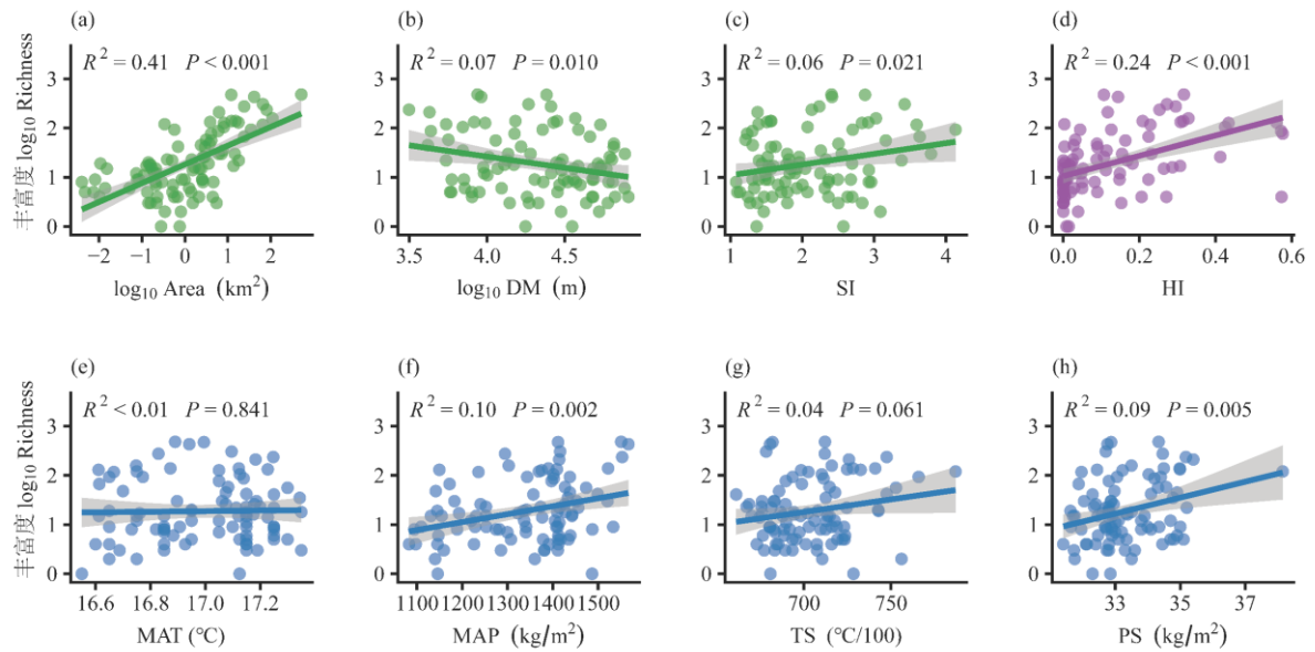
附录 7 草本丰富度与环境因子的相关性。(a)面积(Area);(b)距大陆距离(DM);(c)岛屿形状指数(SI);(d)人类影响指数(HI);(e)年均温(MAT);(f)年降水量(MAP);(g)温度季节性(TS);(h)降水季节性(PS)。
