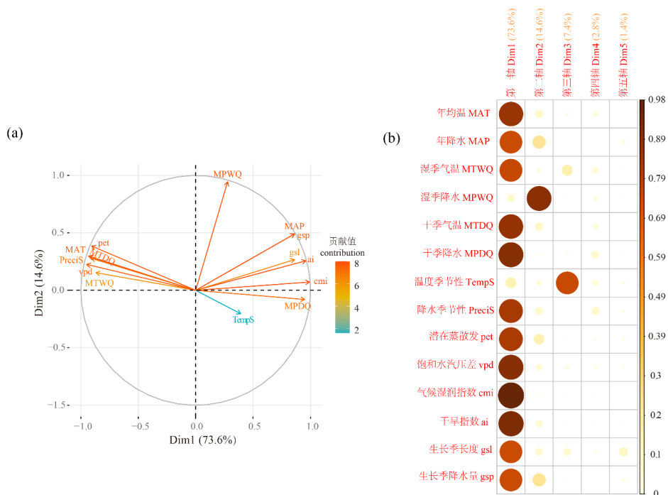
附录 1 本研究气候因子筛选: 主成分分析结果。(a)为主成分分析图;(b)为主成分分析轴的各因子贡献值。
