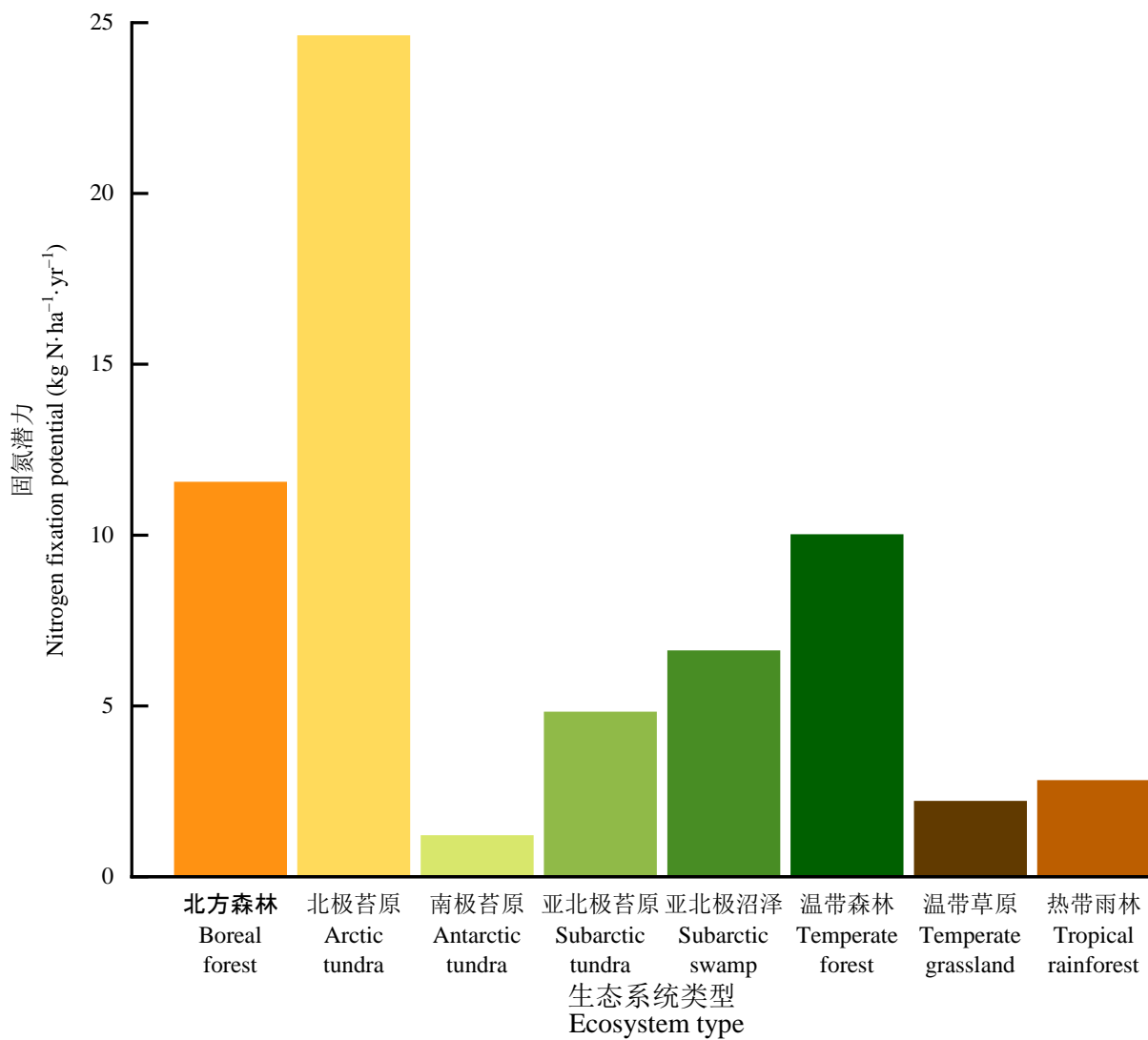
附录5 不同生态系统苔藓-蓝藻共生体固氮潜力多样性
