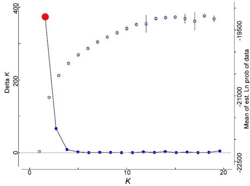
附录6 STRUCTURE分析结果最佳K值的判定。左侧使用Delta K ( \Delta K )方法推断最佳K值, 红色圆点表示最佳K值为2。右侧是数据在不同估计值K下的平均对数似然。
