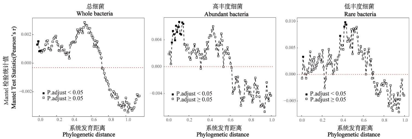
附录 13 细菌最优环境欧氏距离和系统发育距离的 Mantel 相关图。黑色实心点表示多重比较的 Bonferroni 校正后显著相关 ( P < 0.05 )。
