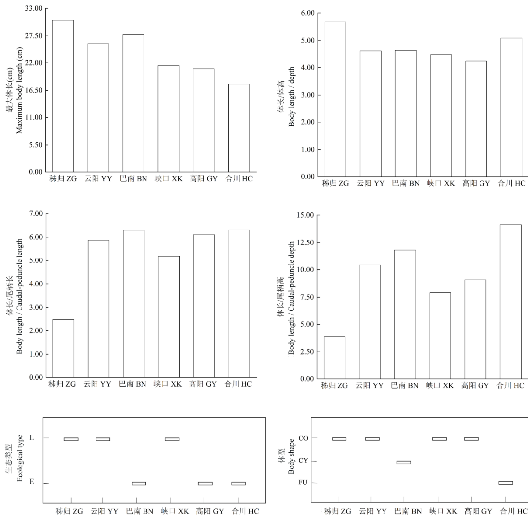
附录3 三峡库区鱼类群落运动功能群落特征加权平均数指数(CWML)空间变化。L: 静水性; E: 广适性; CO: 侧扁形; CY: 圆筒形; FU: 纺锤形。
