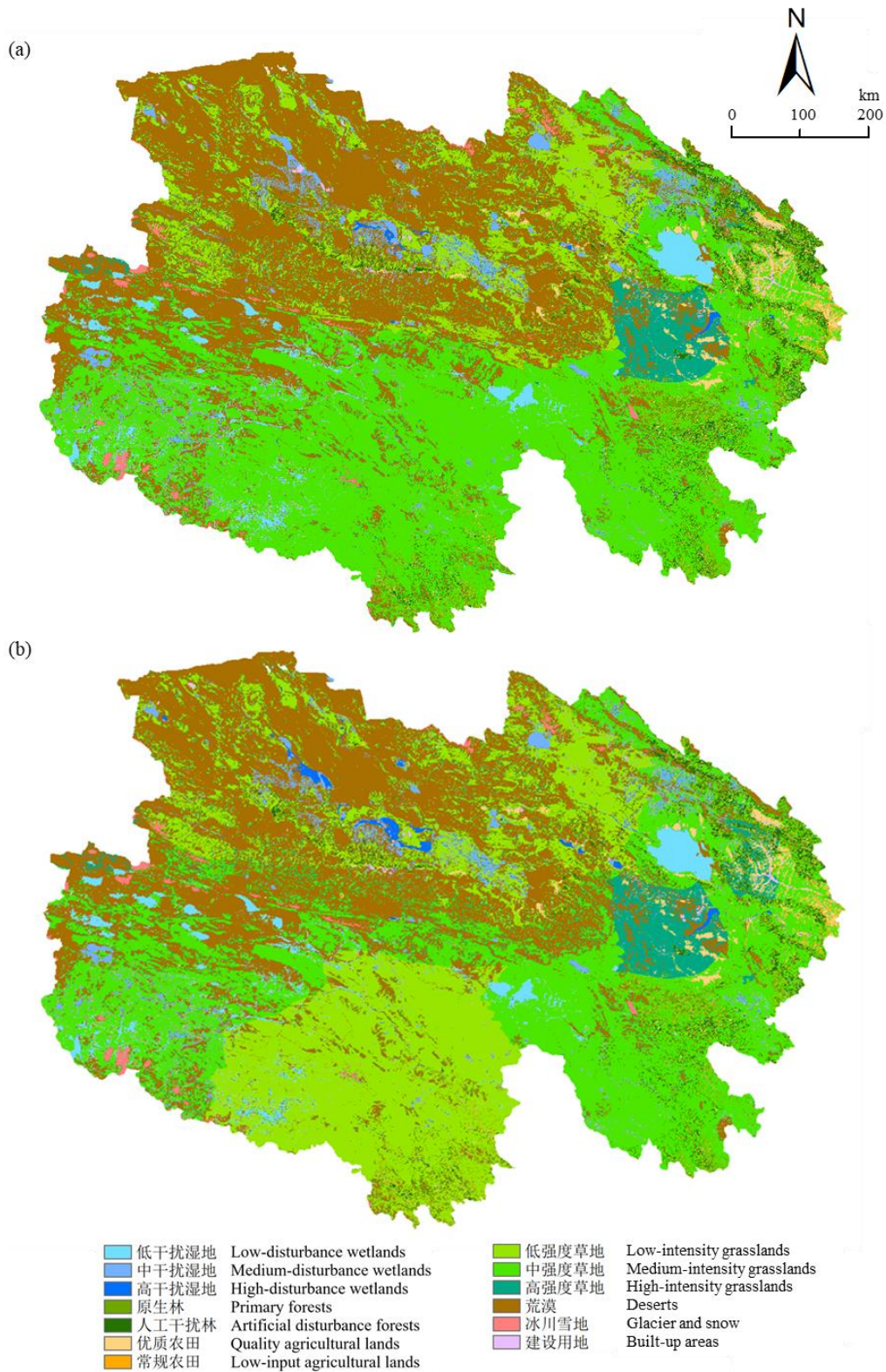
附录 2 青海省 2015 (a)年和 2020 (b)年的土地利用布局。各土地利用类型/干扰强度的描述参见附录 2。 Appendix 2 Land use spatial pattern in Qinghai Province in 2015 (a) and 2020 (b). See Appendix 2 for the description of each land use type/disturbance intensity.
