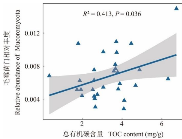
附录11 荒漠土壤毛霉菌门相对丰度与总有机碳含量的关系。 R^2 表示拟合度。
