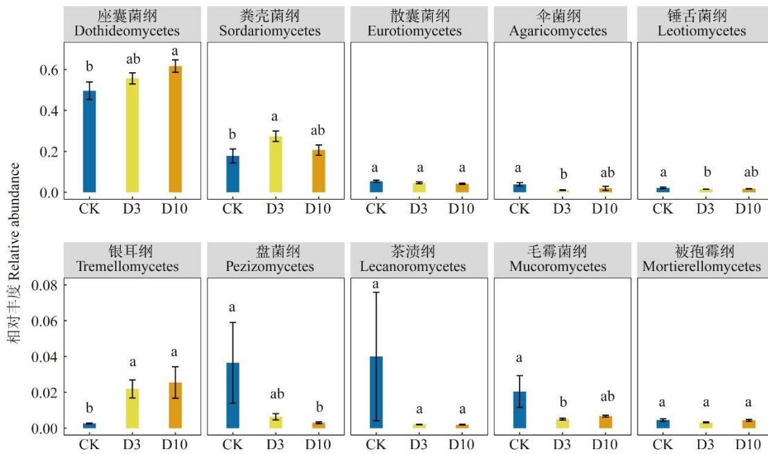
附录 8 荒漠土壤优势真菌纲的相对丰度。CK: 自然对照; D3: 干旱三年; D10: 干旱十年。不同字母表示各优势真菌纲相对丰度在不同干旱处理间的差异显著 ( P < 0.05 ) (nCK = 11, nD3 = 12, nD10 = 11)。
