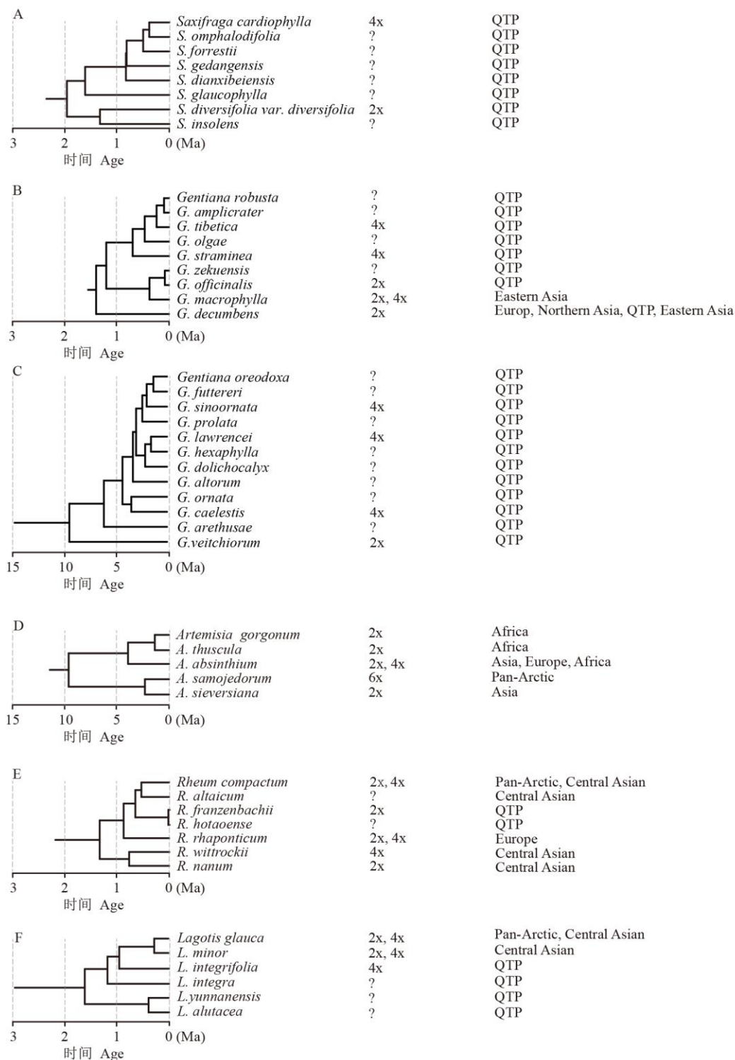
附录3 在系统发育框架下分析植物多倍体的起源。A, 虎耳草属( Saxifraga ), 时间树源自Ebersbach等(2017); B、C, 龙胆属( Gentiana ), 时间树源自Favre等(2016); D, 蒿属( Artemisia ), 时间树源自Tkach等(2008); E, 大黄属( Rheum ), 时间树源自Sun等(2012); F, 兔耳草属( Lagotis ), 时间树源自Li等(2014)。“?”示缺乏染色体数据。
