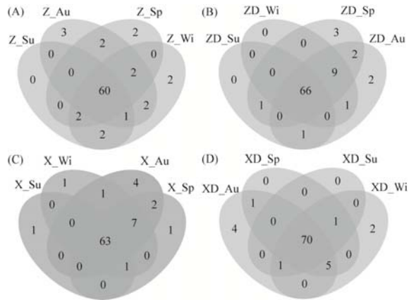
附录3 纲水平下四季土壤样品的Venn图分析。Z: 藻结皮; ZD: 藻结皮下层; X: 藓结皮; XD: 藓结皮下层; Sp: 春天; Su: 夏天; Au: 秋天; Wi: 冬天。
